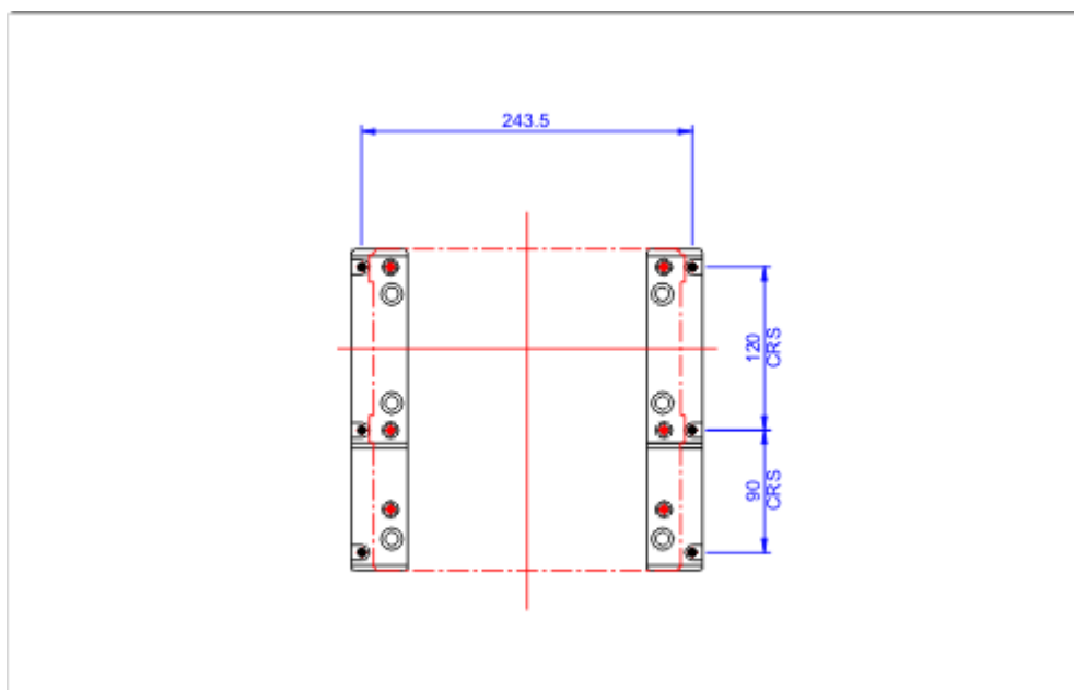
Рисунок 3-2 Габаритные размеры KATflow 150
