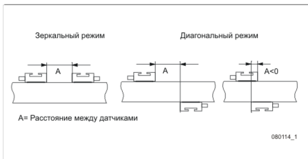
Рисунок 3-4 Конфигурации установки датчиков на трубе
