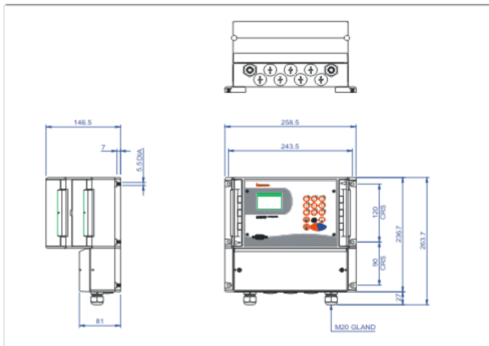
Рисунок 3-2 Габаритные размеры KATflow 150
